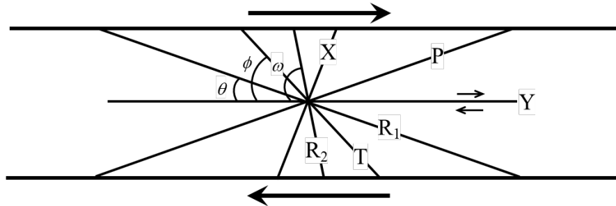
図2 剪断帯に垂直で剪断方向に平行な面で描いた模式図
